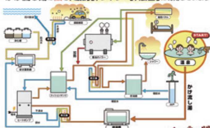
(上図) ヒートポンプシステムの概要図
